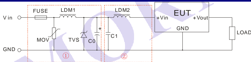
(图 1) EMC 推荐电路
