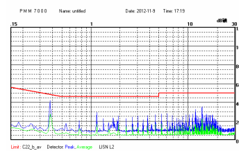
K78L05-1000R2 传导测试效果图 (负线)
