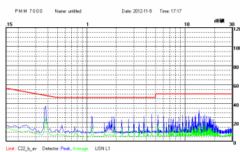
K78L05-1000R2 传导测试效果图 (正线)
